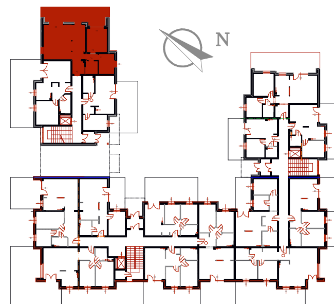
Rzut parteru
