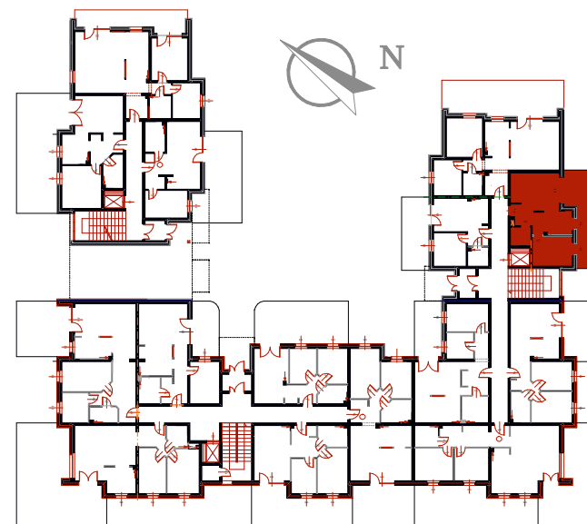
Rzut parteru
